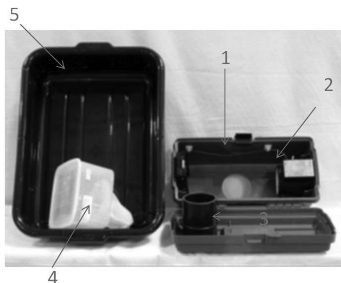
Figura 2: trappola tipo Gravid non assemblata.
