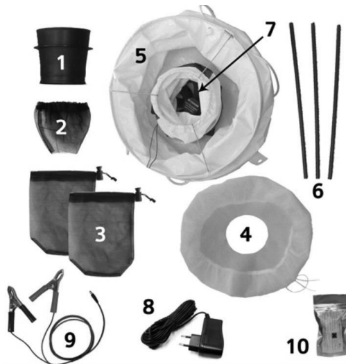
Figura 6: trappola BG-Sentinel non assemblata.
